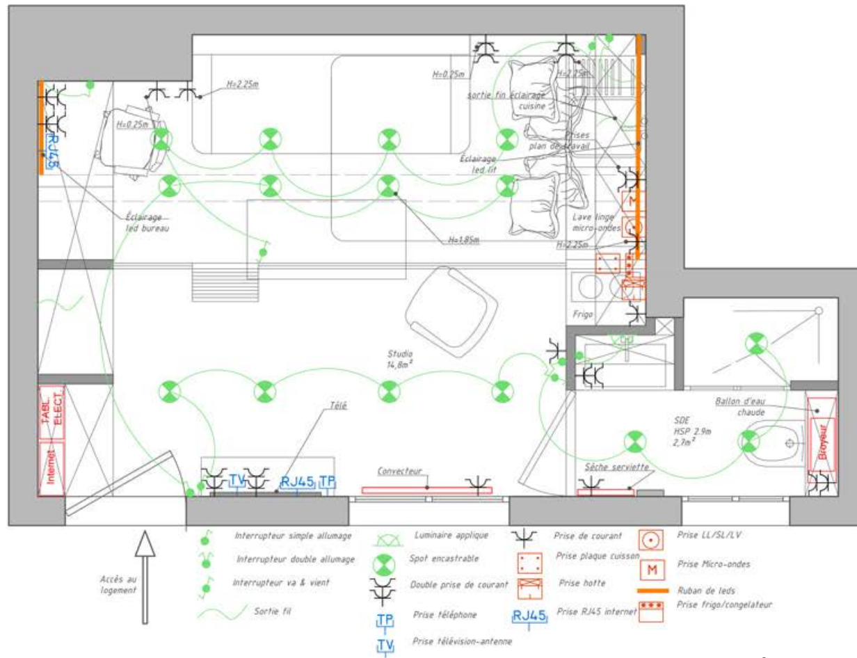
Plan électrique
