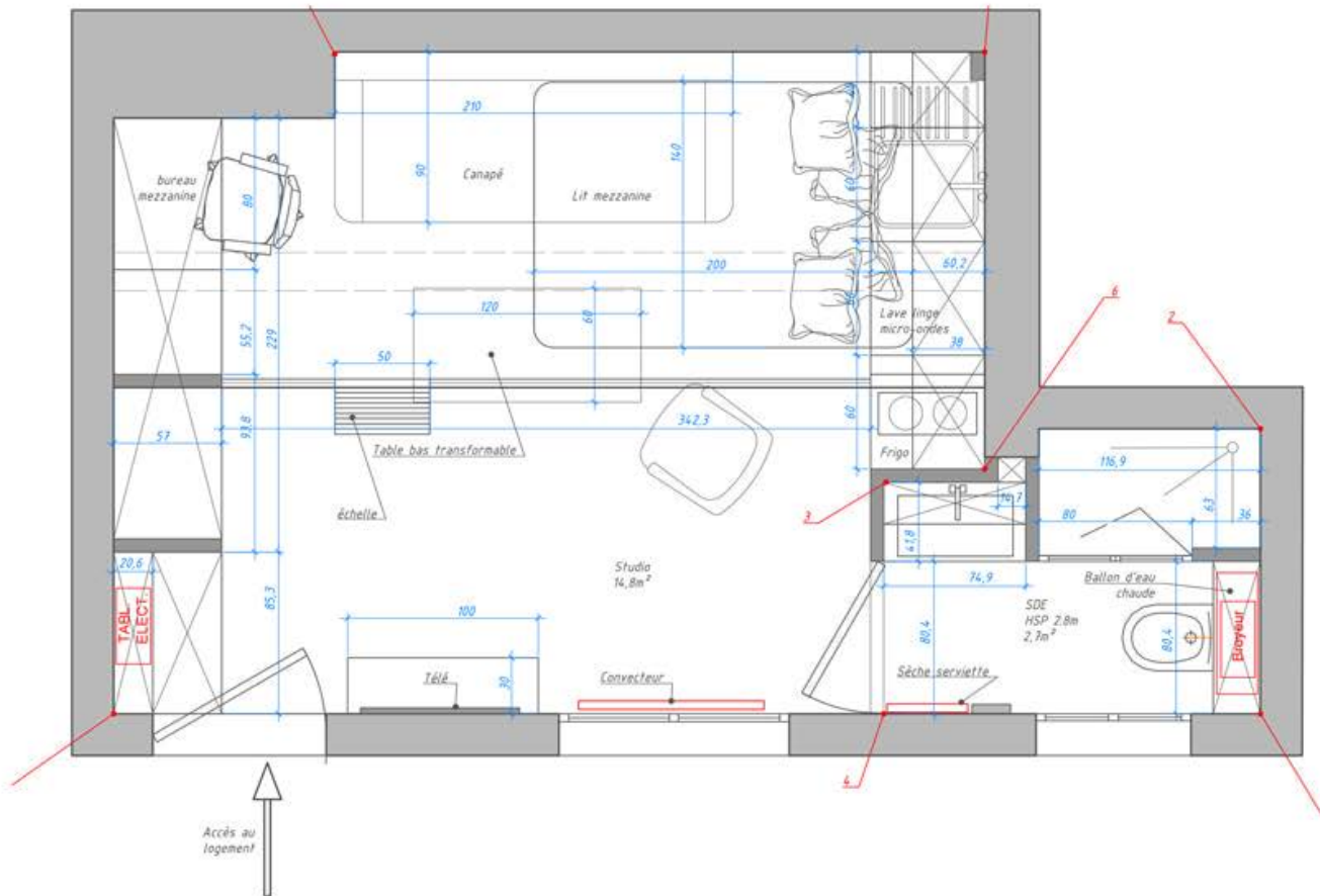
Plan projeté
