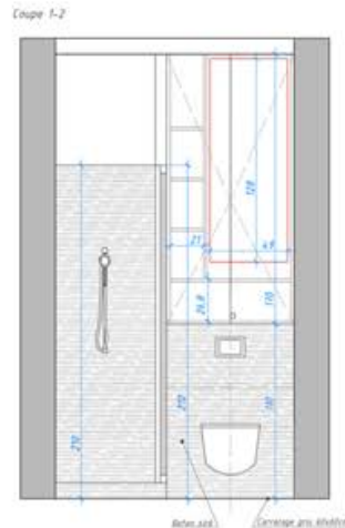
Coupes SDB
