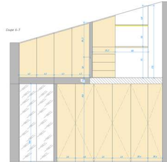
Coupe bureau
