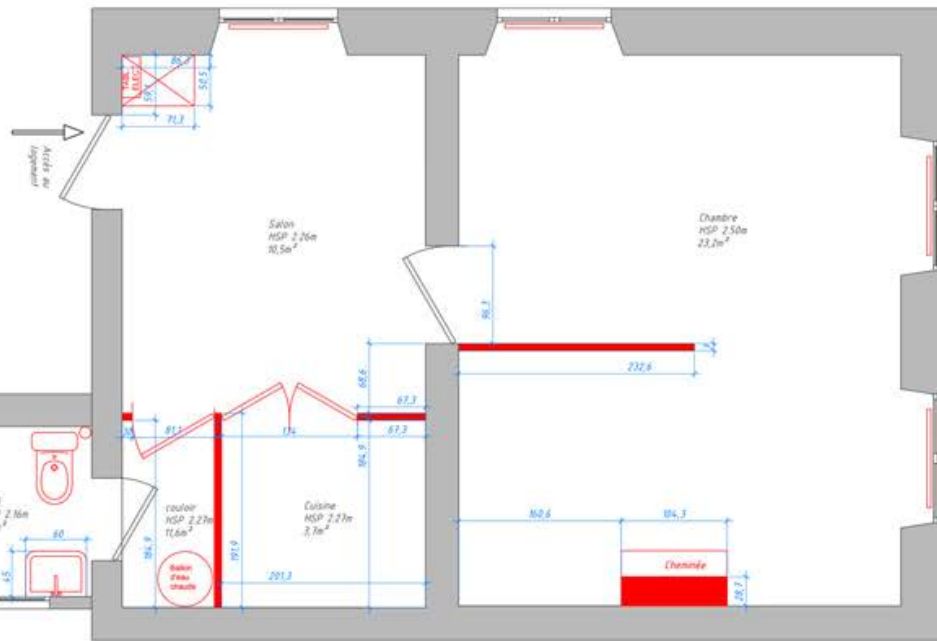
Plan démolition
