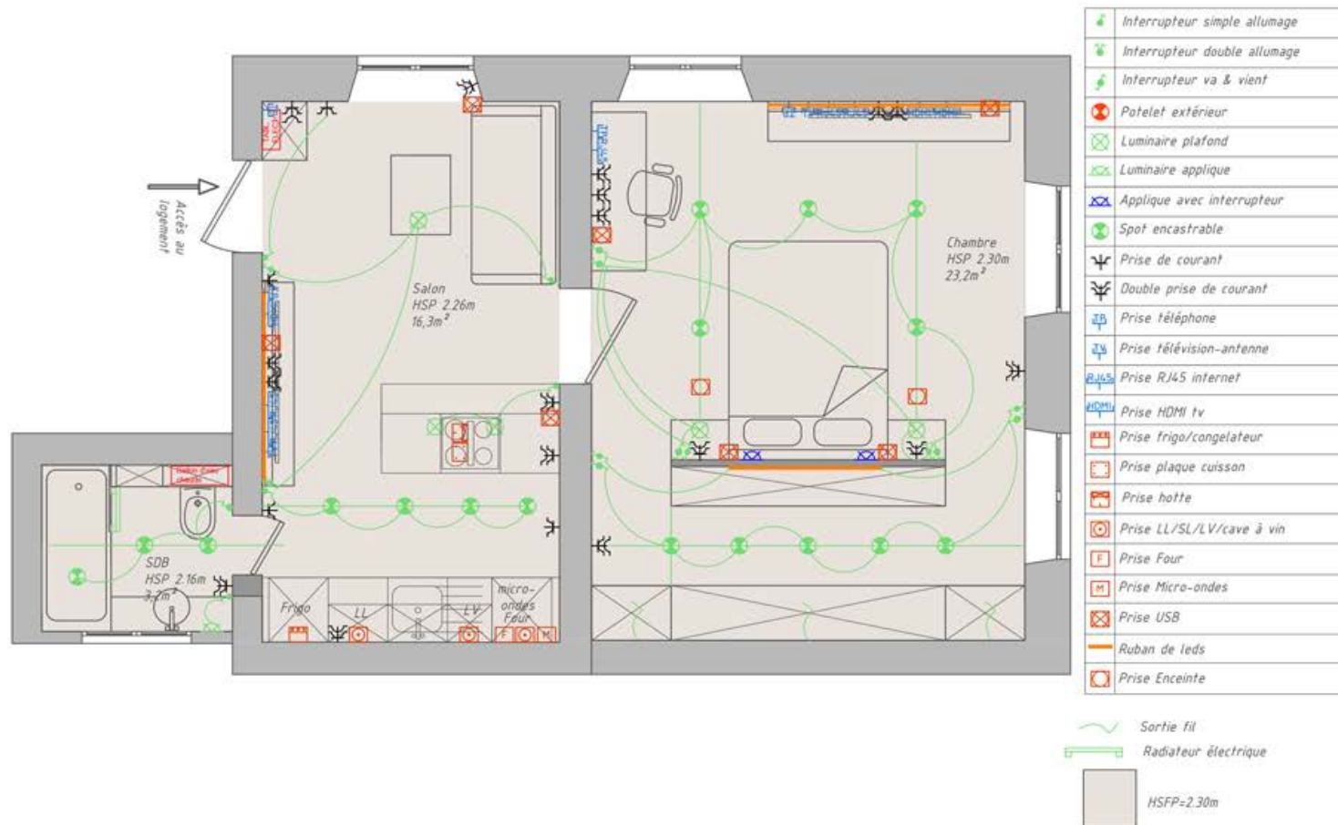
Plan électrique
