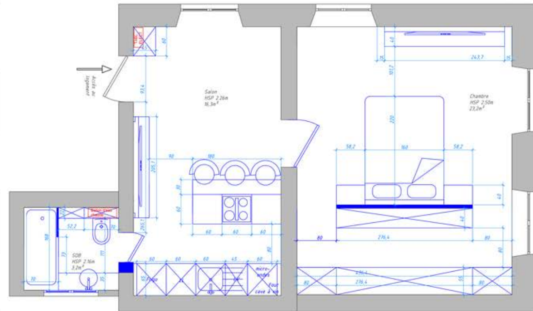
Plan maçonnerie
