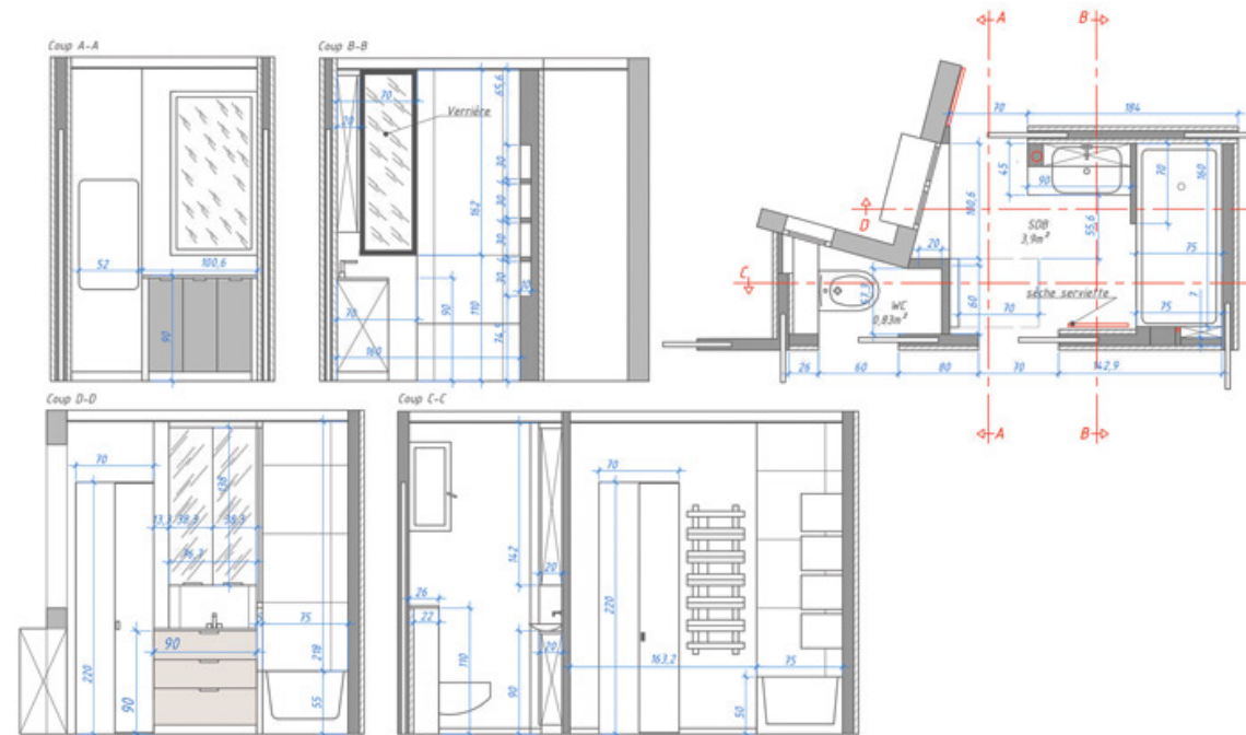
Coupes SDB
