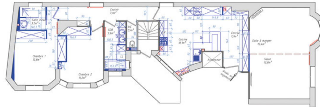
Plan maçonnerie
