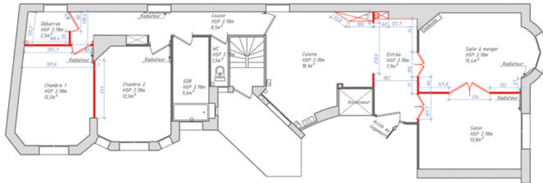
Plan démolition
