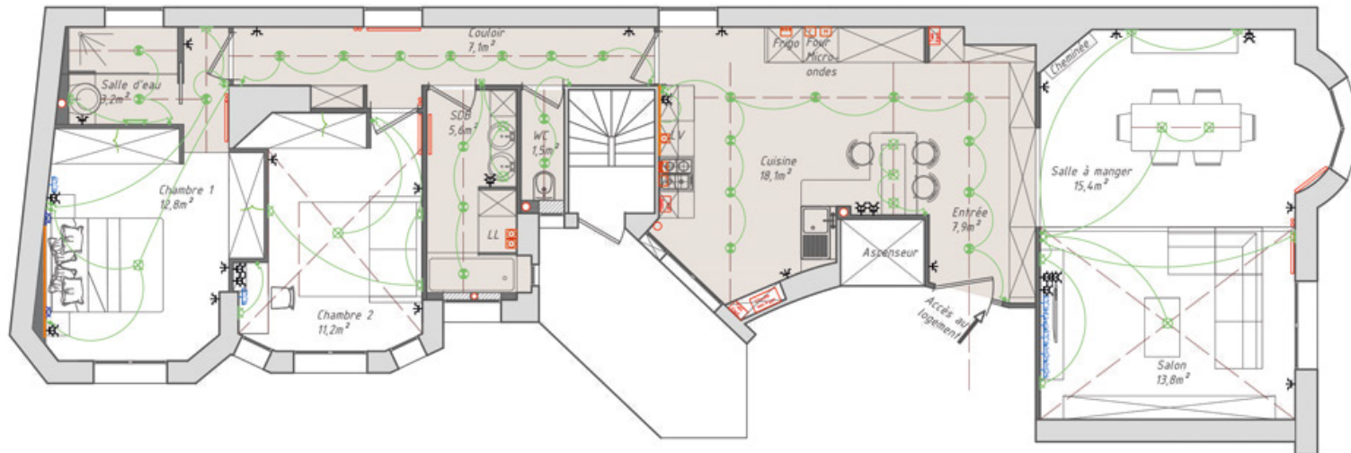
Plan électrique
