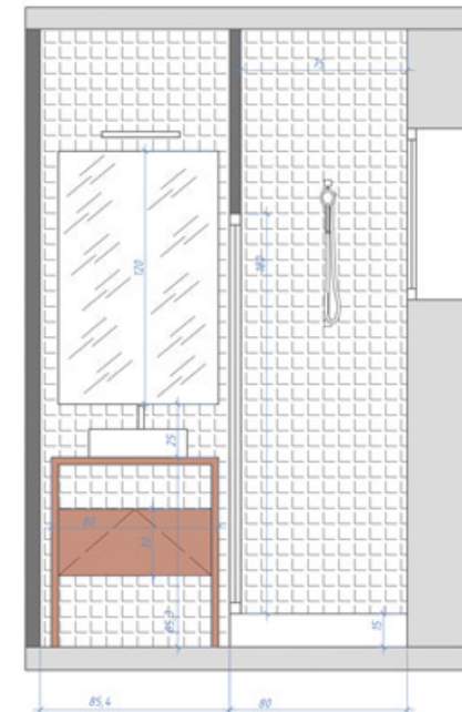
Coupes SDB
