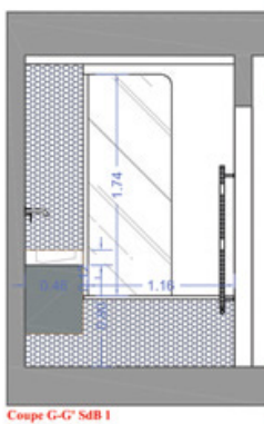
Coupe G-G' SdB 1
