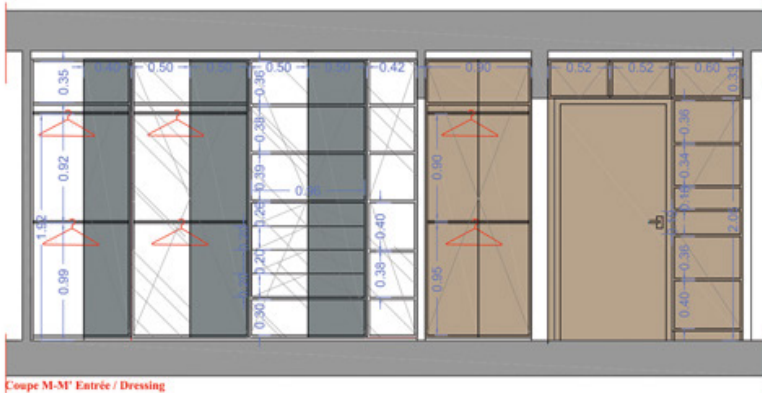
Coupe M-M' Entrée / Dressing
