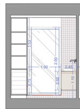
Coupe L-L' SdB 2
