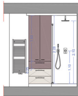
Coupe K-K' SdB 2
