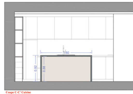
Coupe C-C' Cuisine
