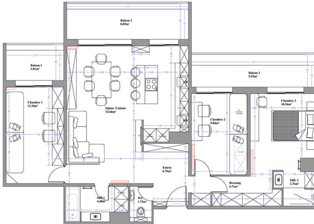
Plan projeté
