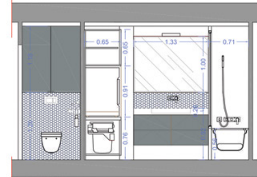
Coupe F-F' WC / SdB 1
