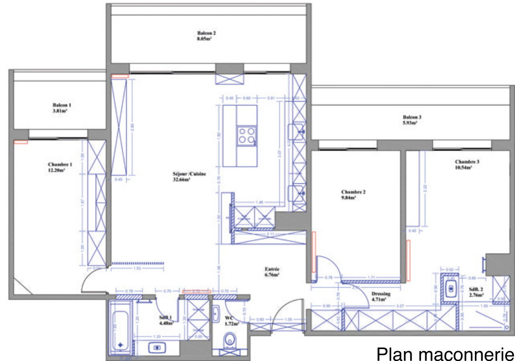
Plan démolition
