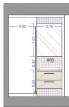
Coupe J-J' SdB 2
