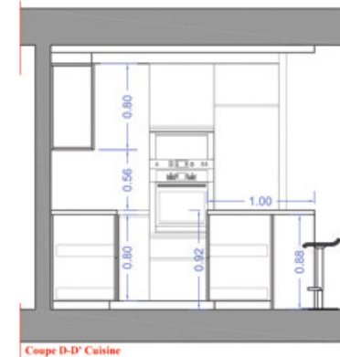
Coupe D-D' Cuisine
