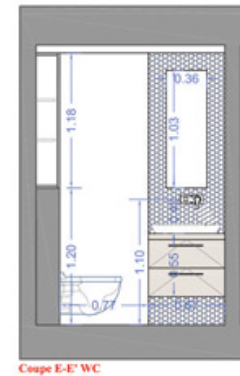
Coupe E-E' WC
