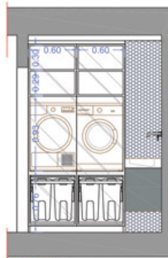
Coupe H-H' SdB 1
