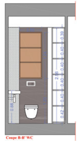
Coupes WC
