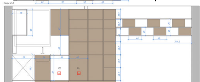
Coupes cuisine
