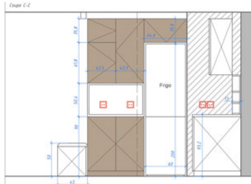
Coupes cuisine
