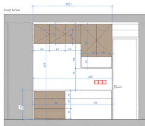
Coupes dressing
