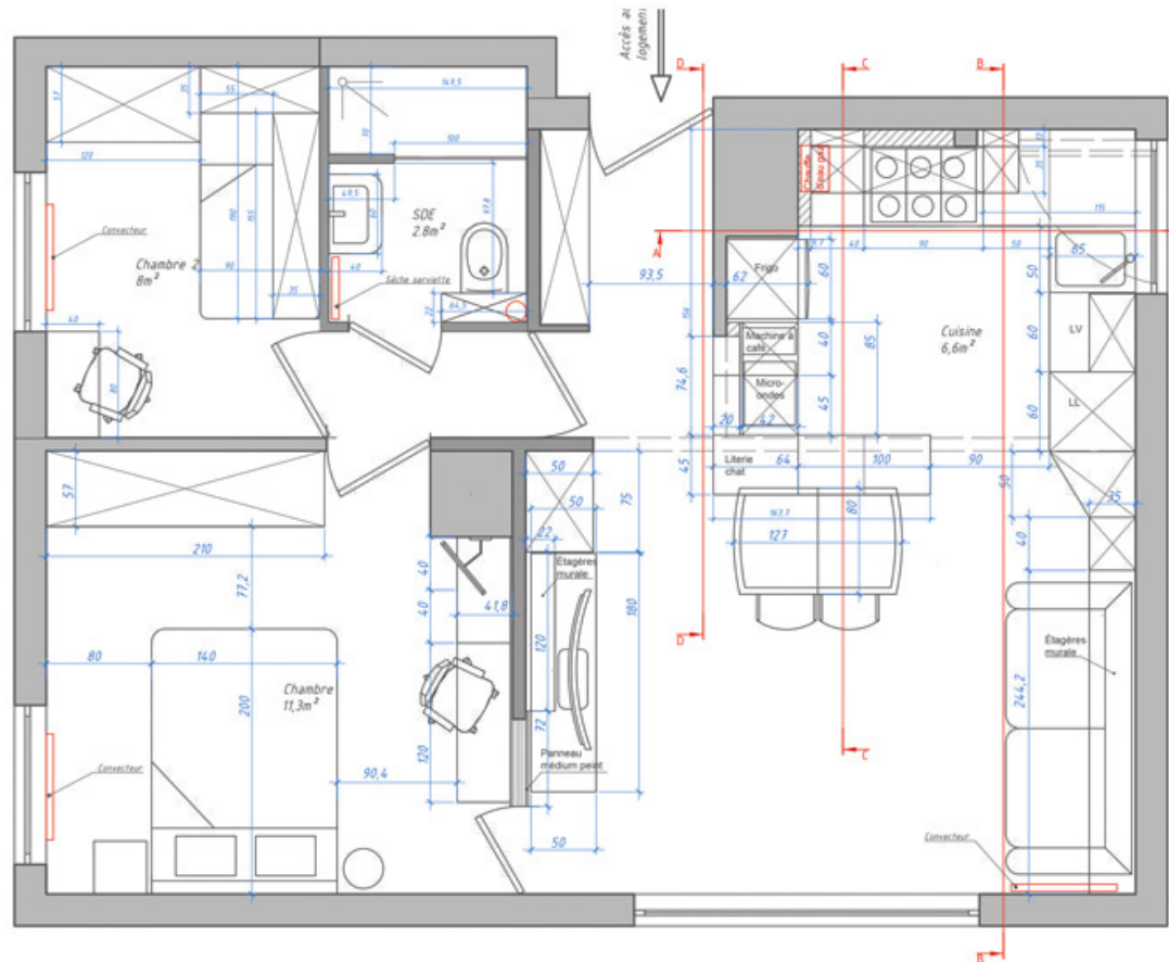
Plan projeté
