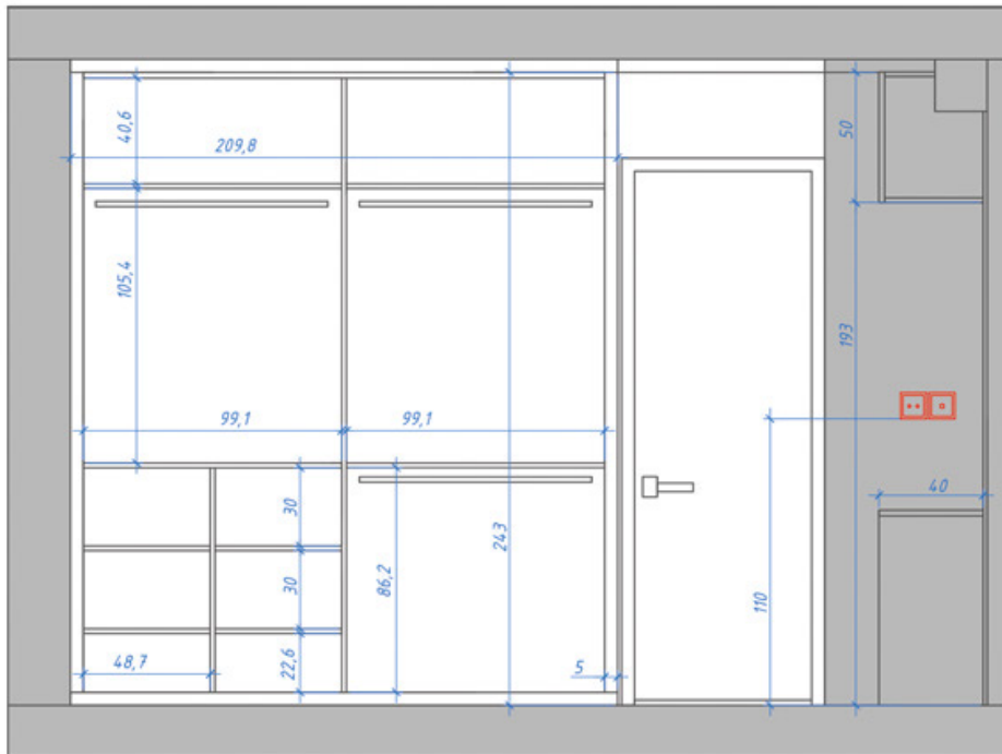
Coupe armoire
