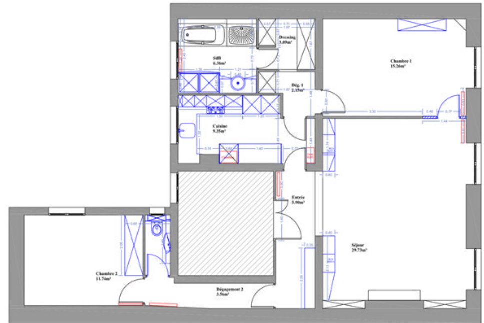
Plan maçonnerie
