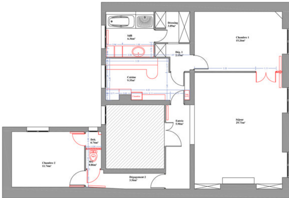
Plan démolition
