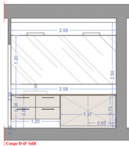
Coupe D-D' SdB
