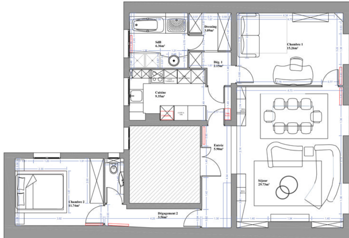
Plan projeté
