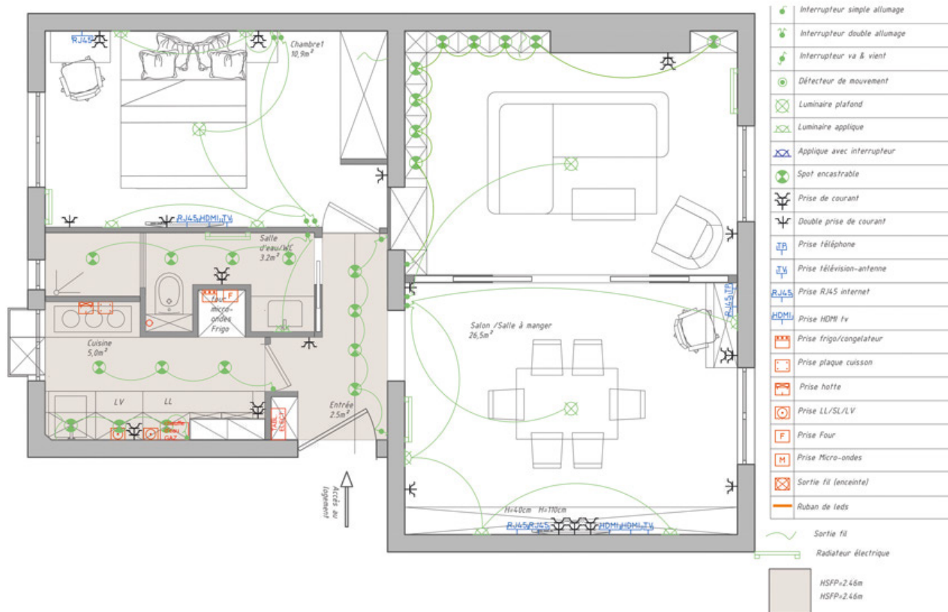
Plan électrique
