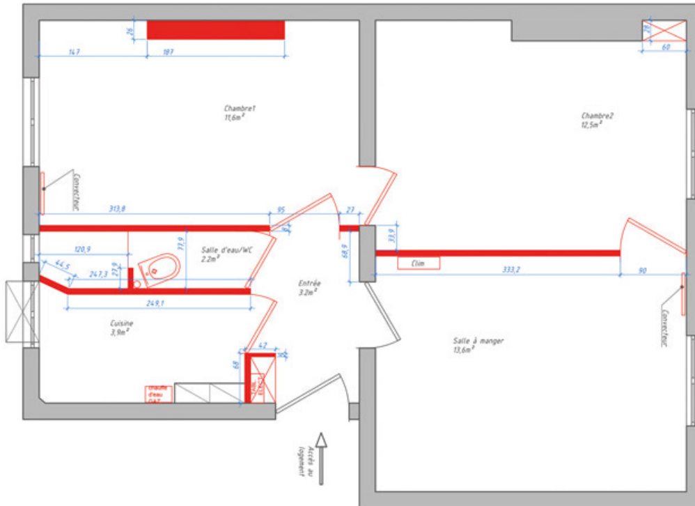
Plan démolition
