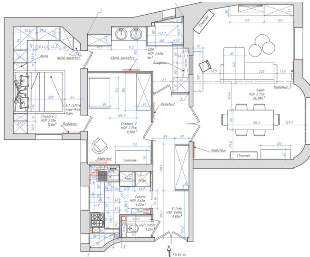
Plan projeté
