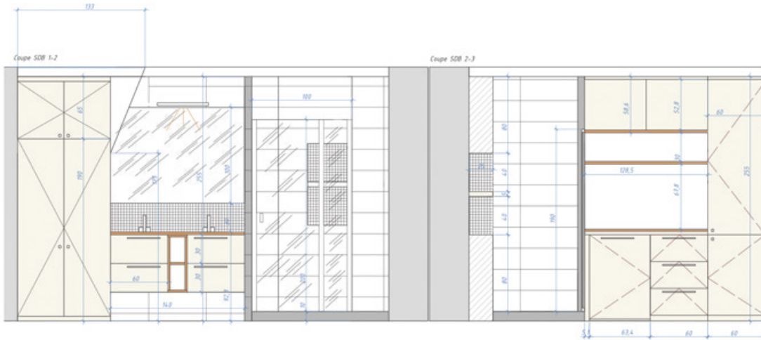
Coupes SDB
