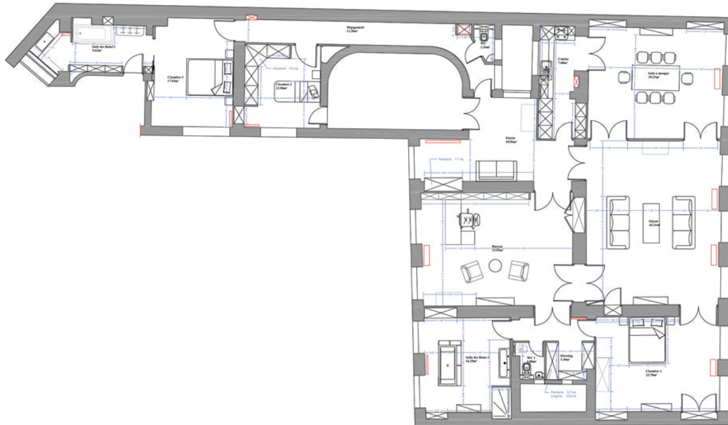
Plan projeté
