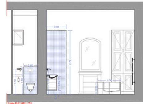
Coupes SDB
